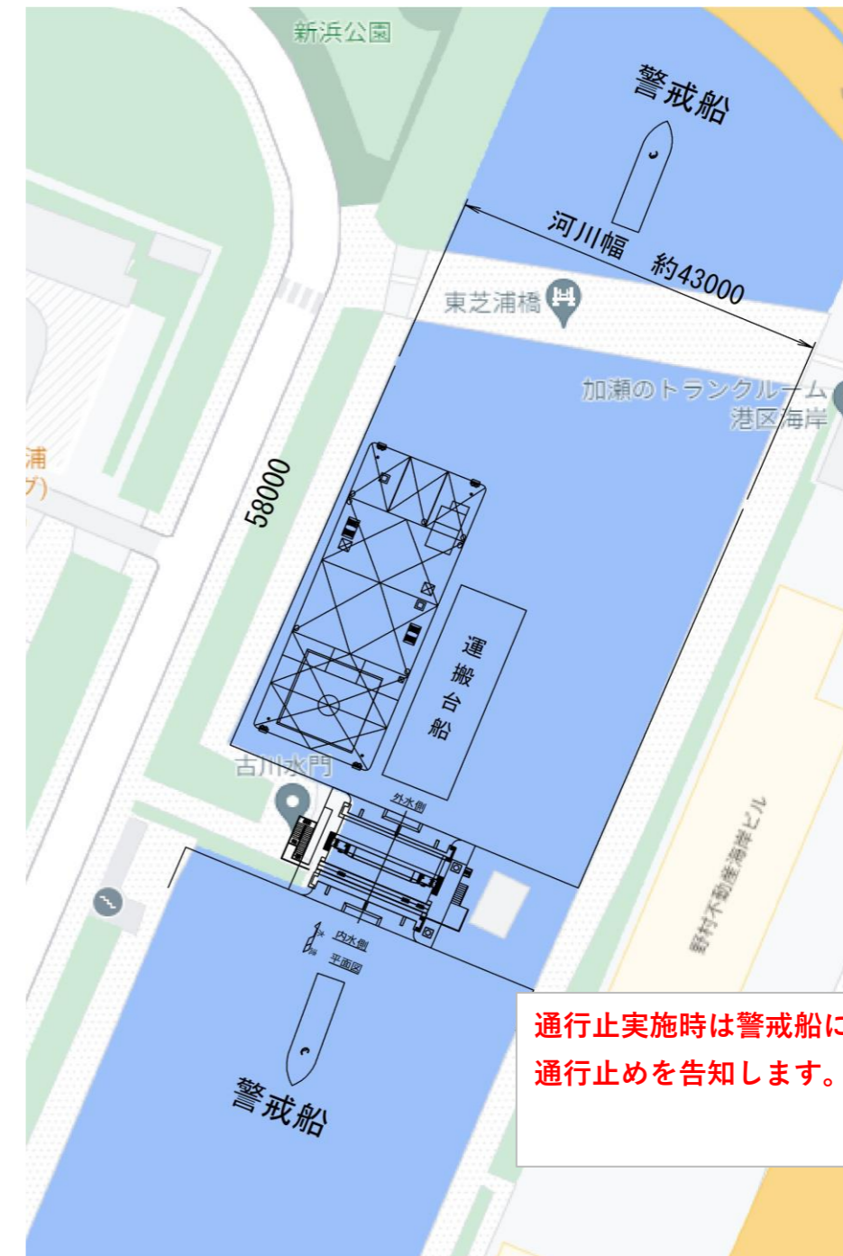
作業時の船舶配置図
