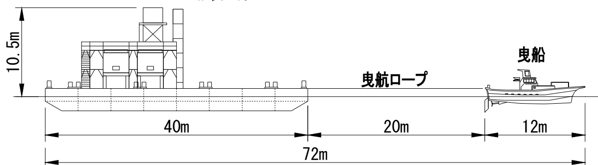
アスファルトクッカー-艀装台船
