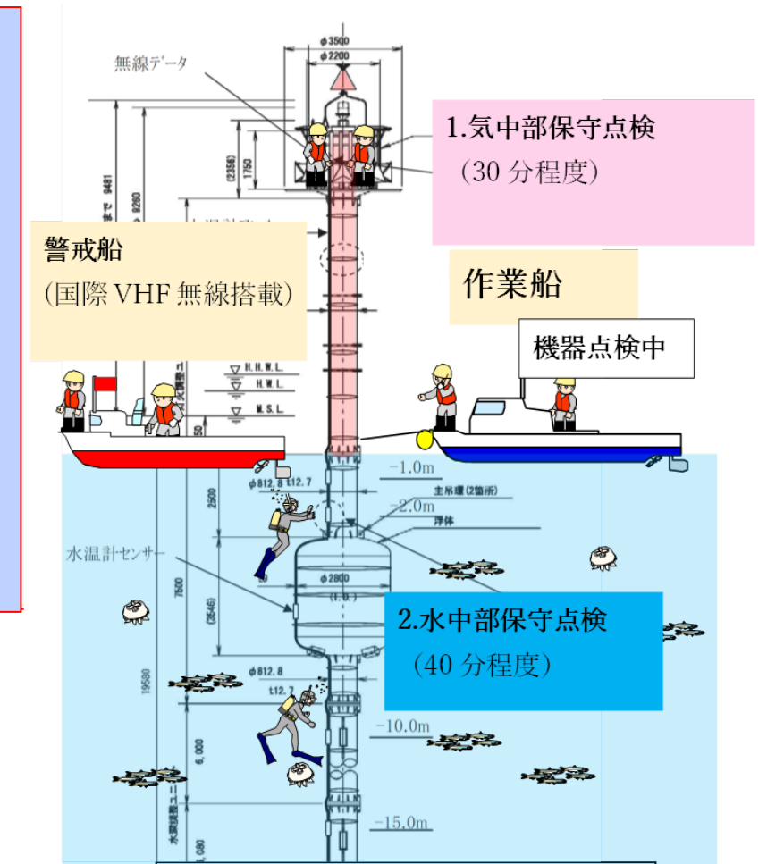
図-3 気中部点検作業状況図
