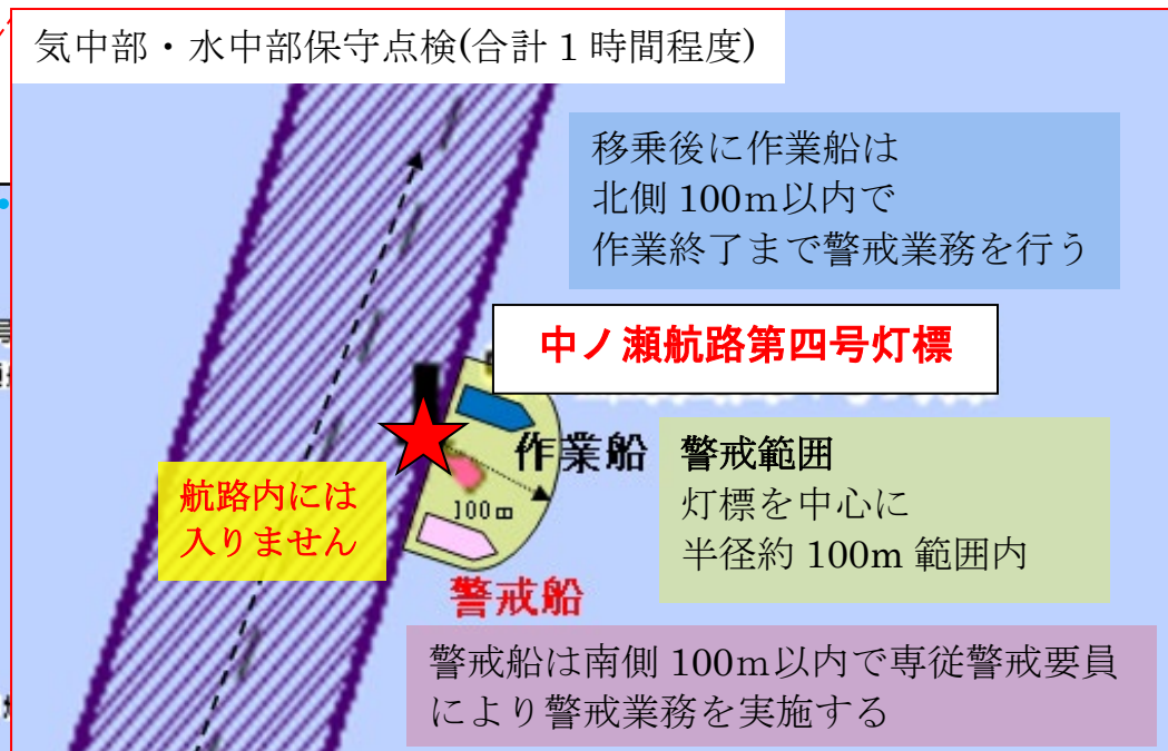
図-2 作業船・警戒船配置図
